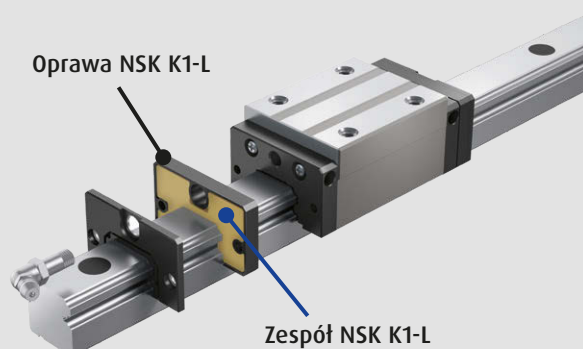
Zaawansowany zespół smarujący NSK K1-L
