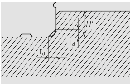
Rys. 9. Odsadzenie dla powierzchni odniesienia szyny
