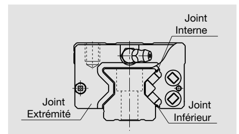
Fig. 10 Vue de la glissière à rouleaux équipée des pièces d'étanchéité à la poussière
