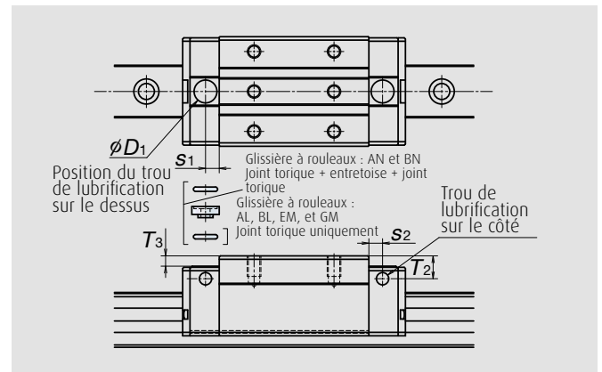
Fig. 8 Positions des trous de lubrification en haut et sur le côté
