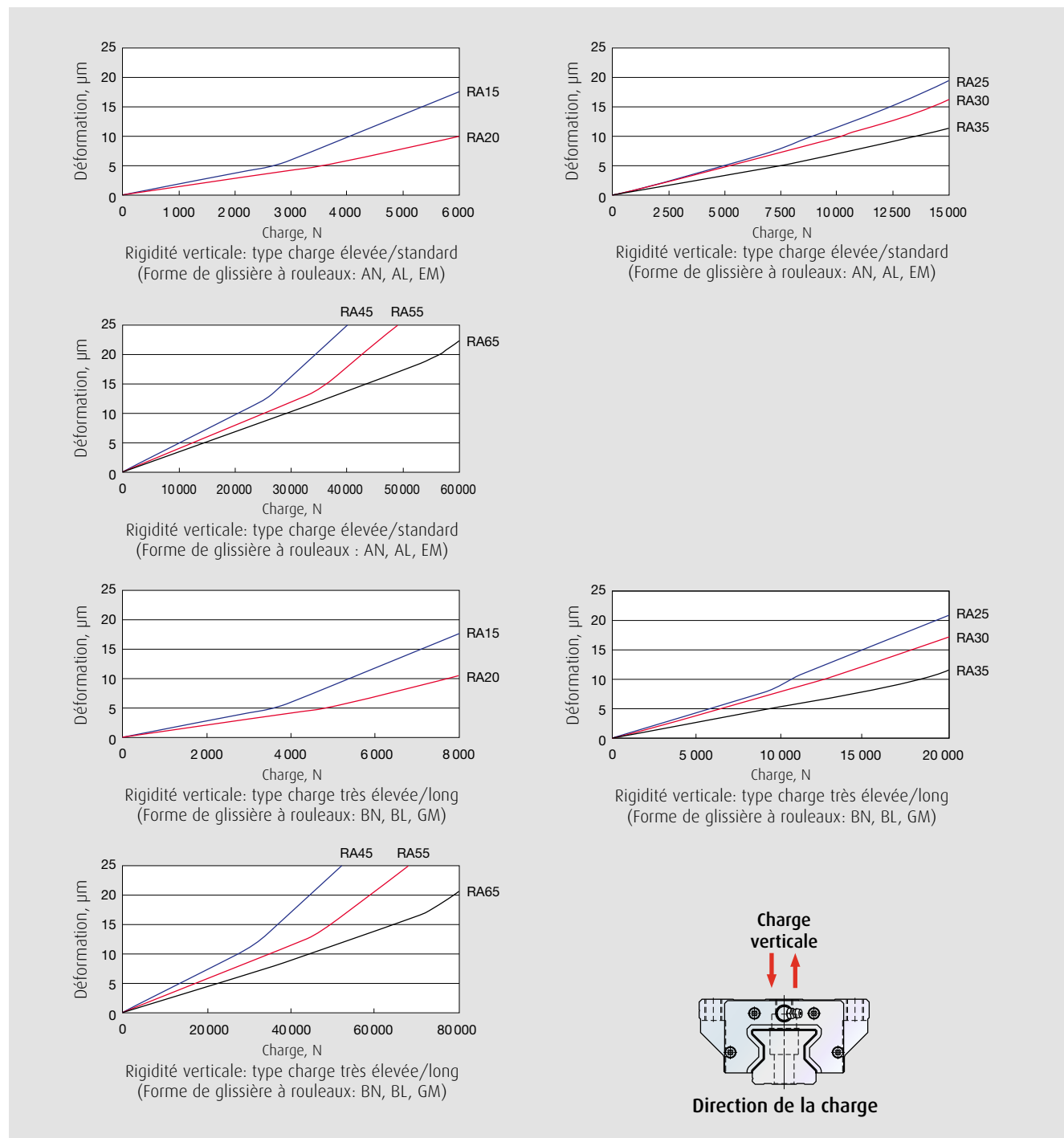
Fig. 5 Courbe de rigidité théorique dans la direction verticale
