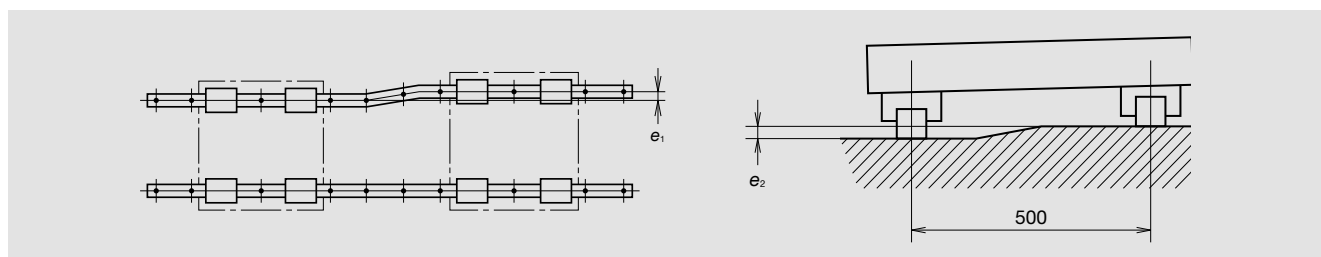
Fig. 15 Tolérance d'installation
