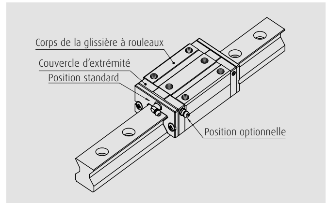
Fig. 7 Position de montage des accessoires de lubrification
