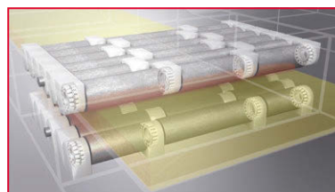
Rollensegmenteinheit
